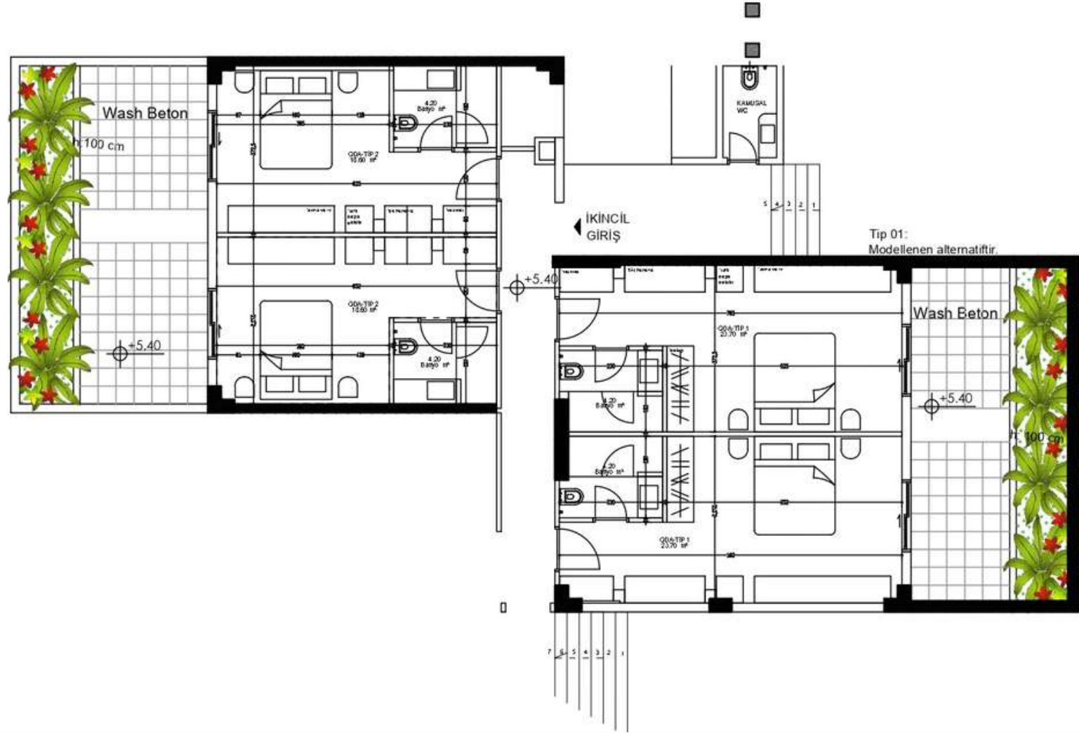
BODRUM KAT MİSAFİR ODASI PLANI 35M2
